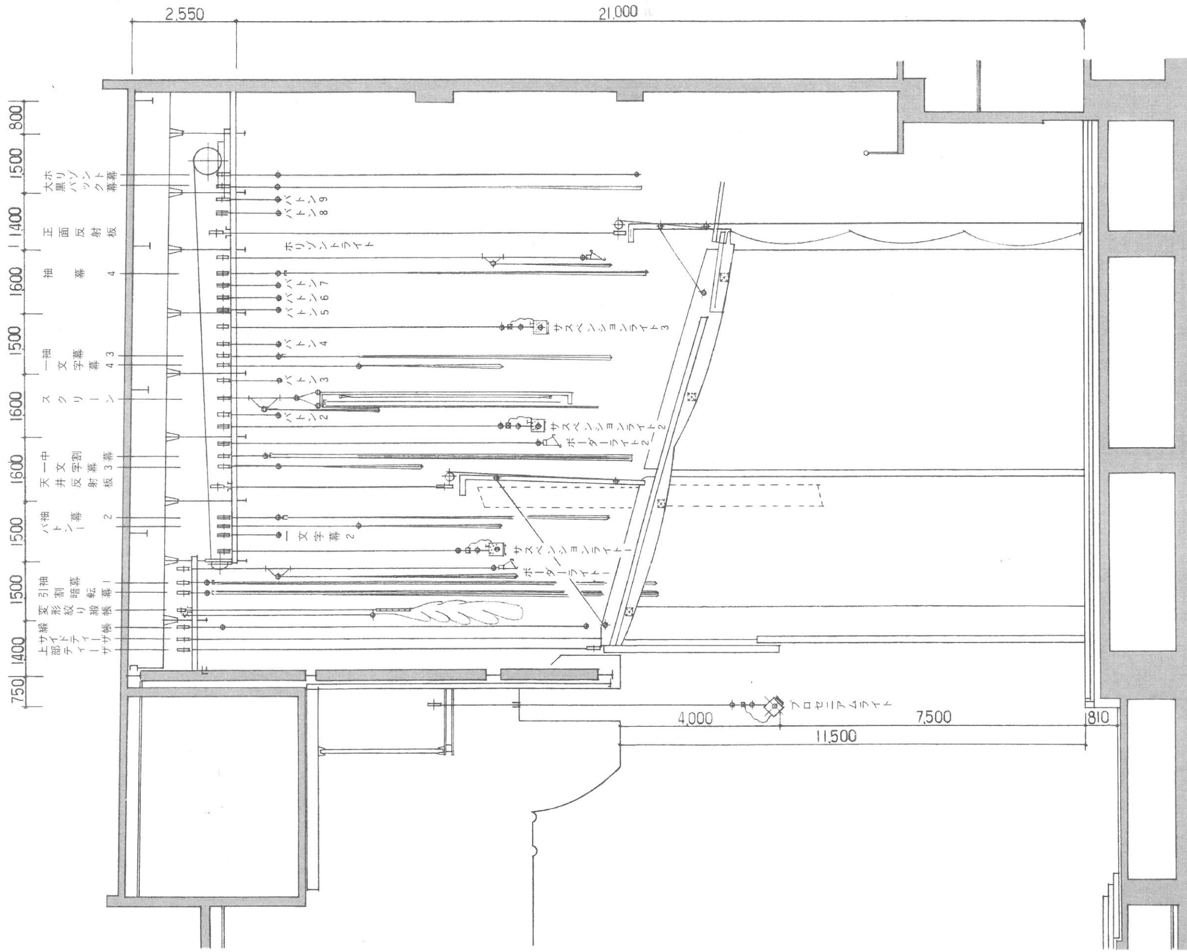
西条市総合文化会館 大ホール舞台断面図
